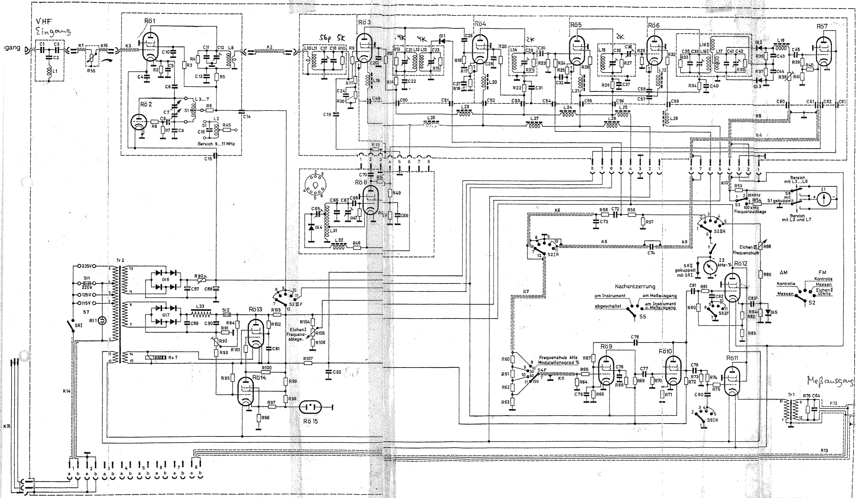
Stromlauf FREQUENZHUBMESSER Type FMV BN 4620
