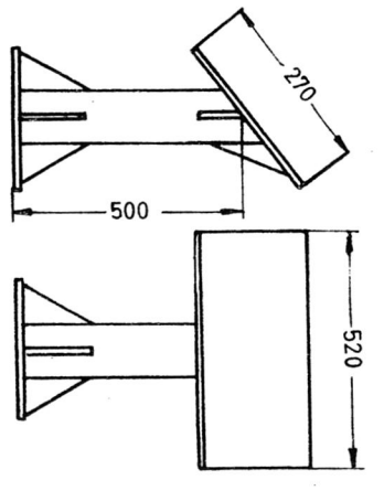
Empfänger - Konsole
