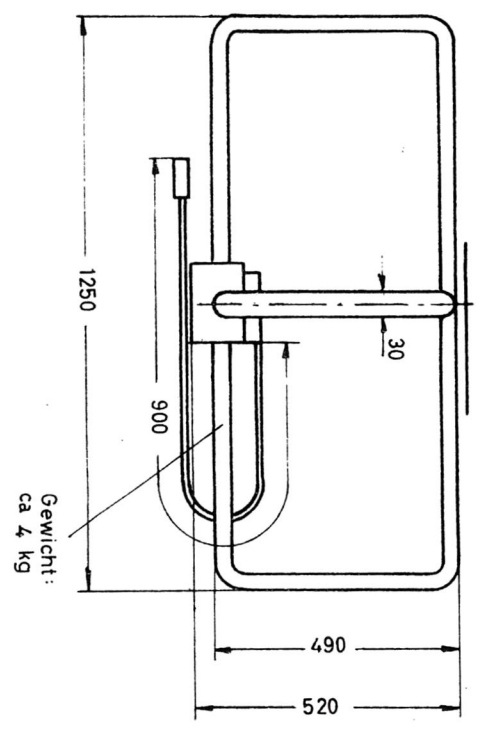
Luft-Kreuzrahmen Typ PR 310/S
