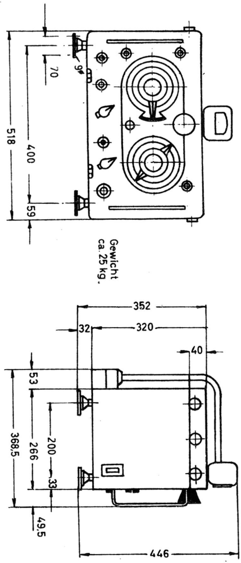
Empfänger Typ PE 398
