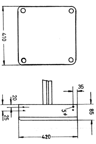
Ferrit - Kreuzrahmen
