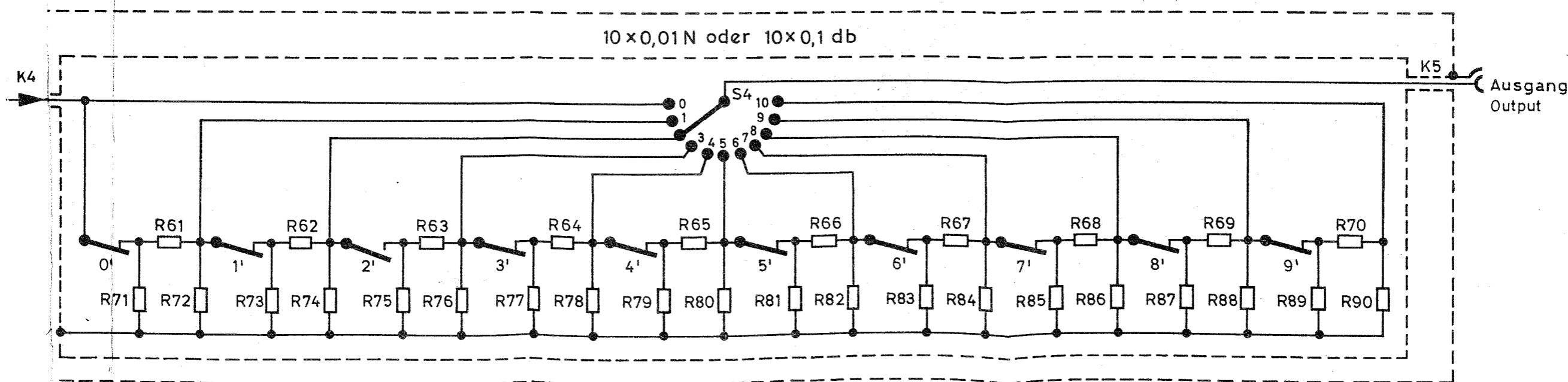
Stromlauf Circuit Diagram
