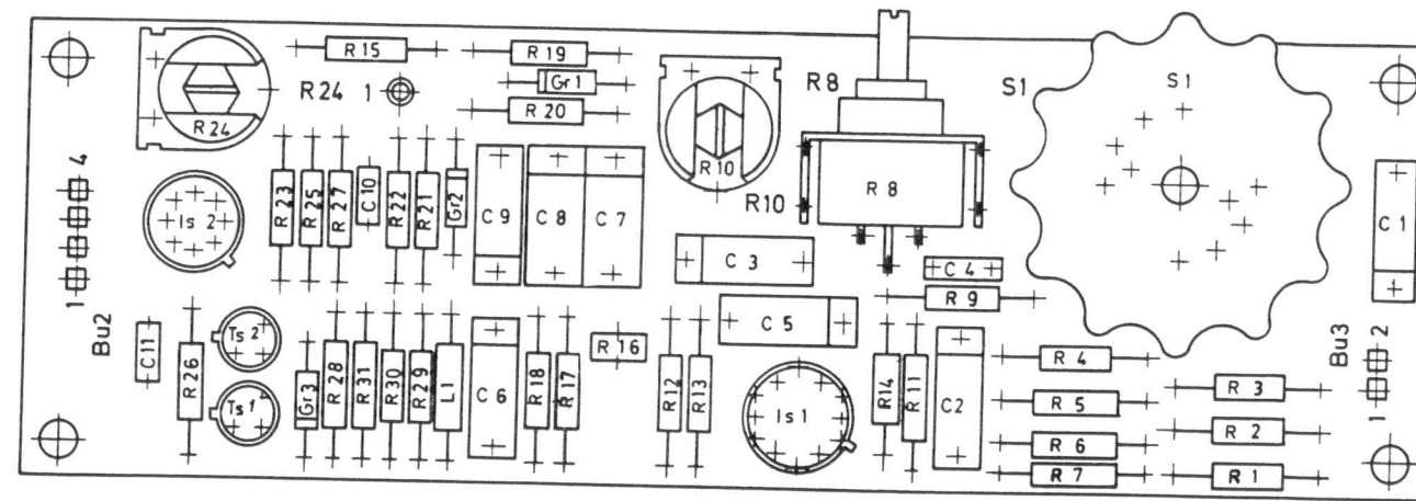
Bestückungsplan Breitbandverstärker Printed Circuit Board Wide-Band Amplifier
