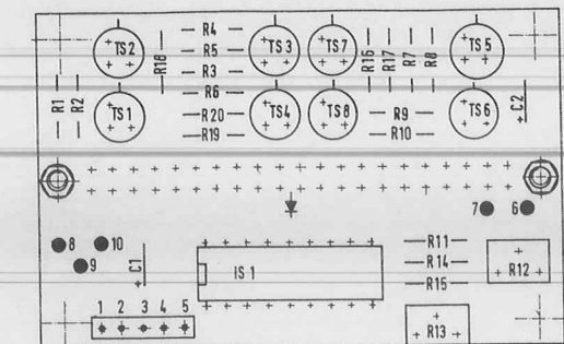
Abstimmmanzeige 52.1703.070.00 (02)
