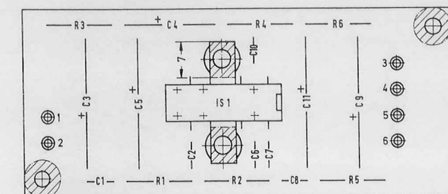
NF-Verstärker 52.1800.150.00 (02)
