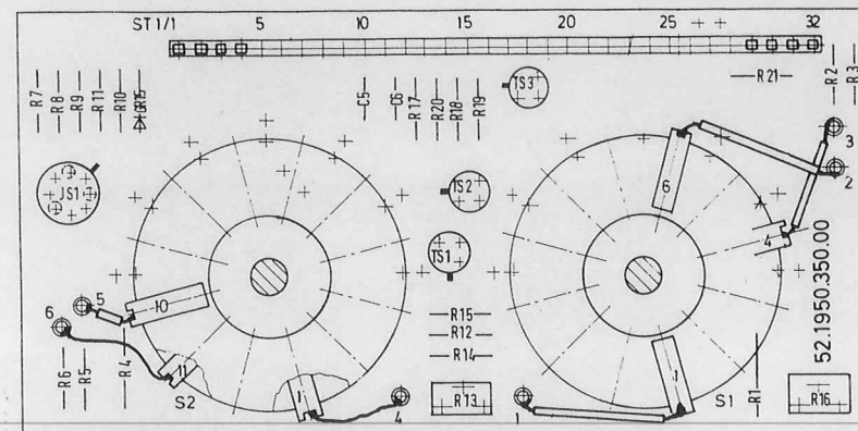
Wahlschalter 52.1950.350.00 (04)
