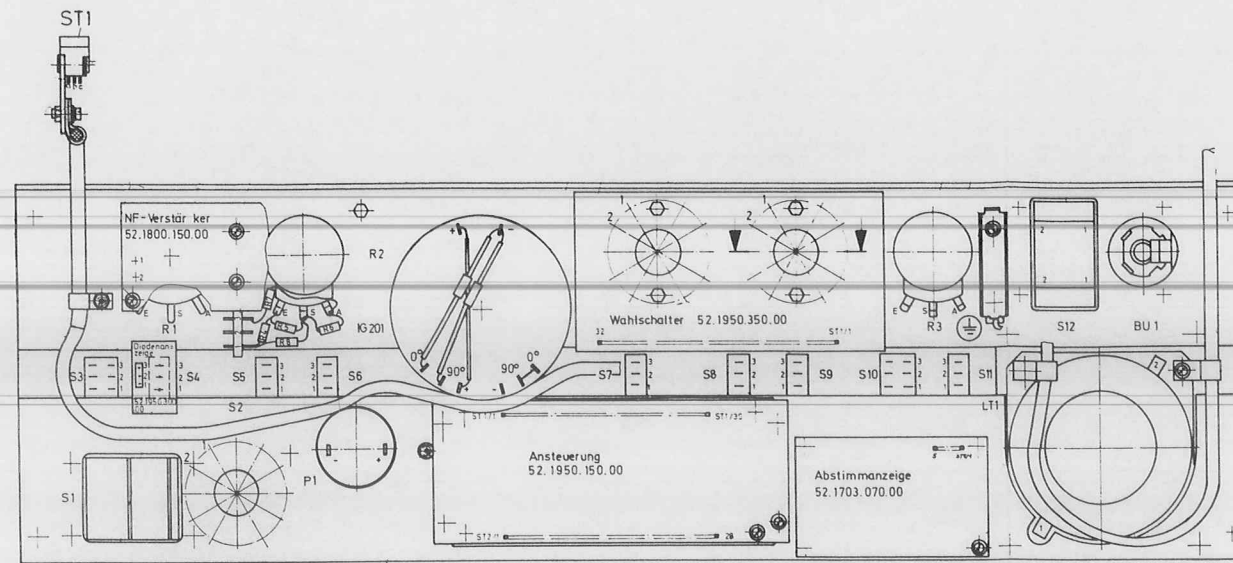
Chassis 52.1950.025.00 (—)
