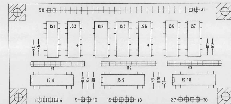
Ziffermanzeige 52.1950.100.00 (01)
