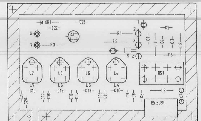
Eingangsfiler 52.1822.100.00 (-)
