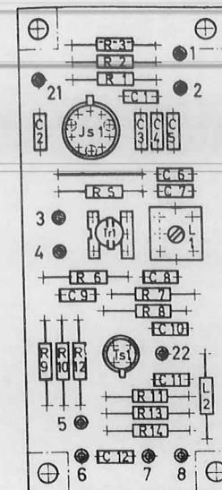
Trennverstärker 2 52.1363.550.00 (03)
