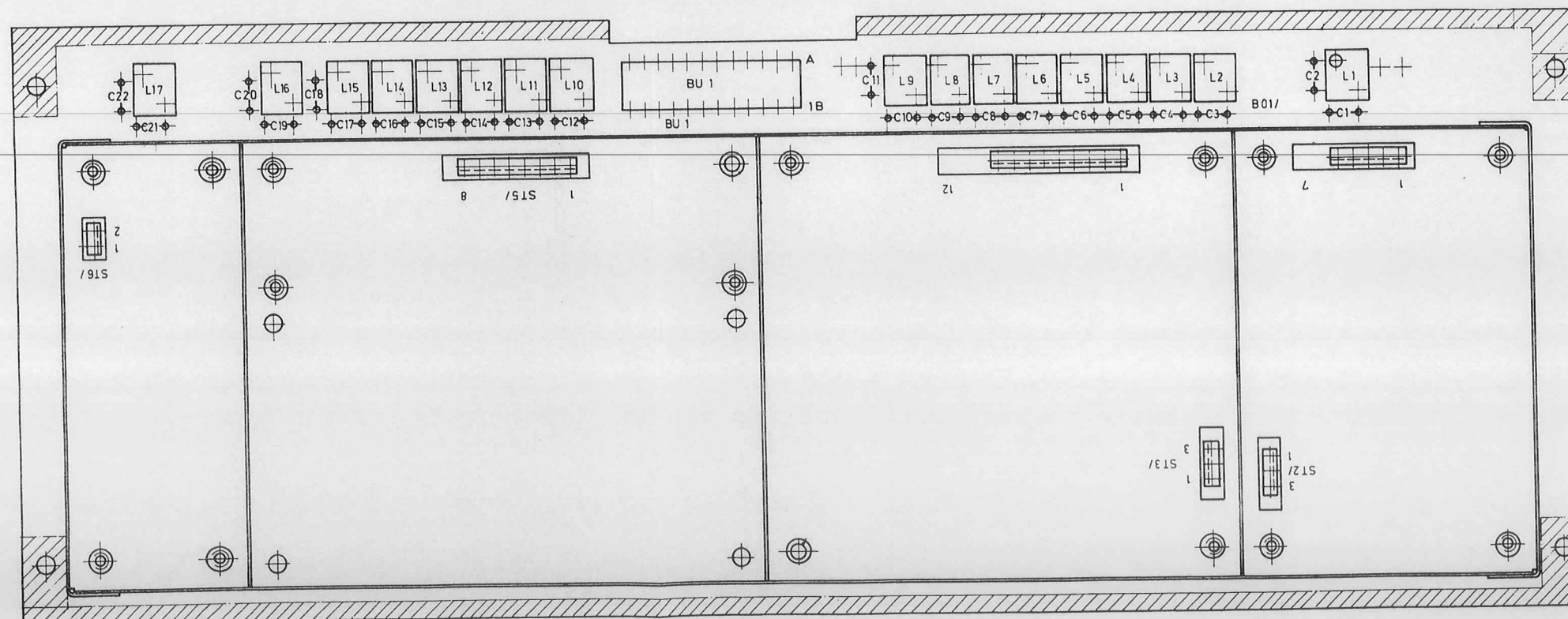
Grundkarte 1. Oszillator 52.1821.101.00 (02)
