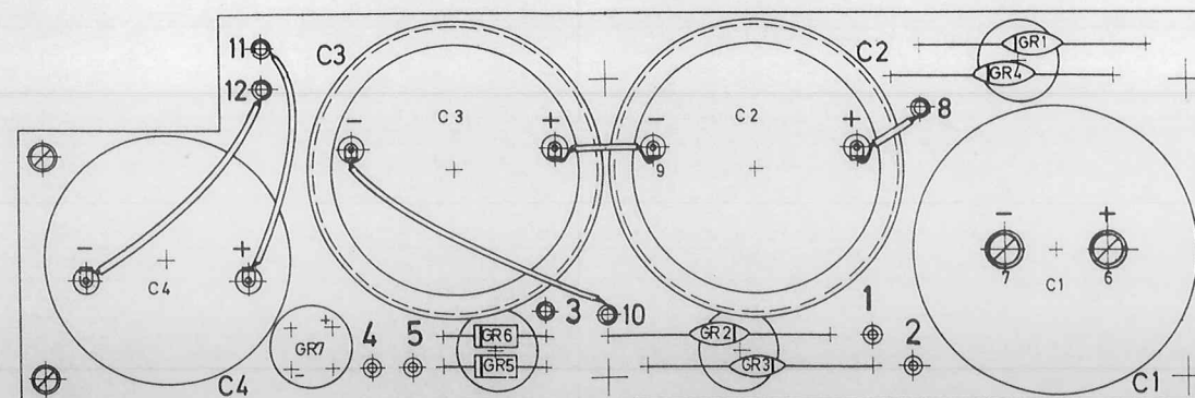
Elko-Aufbau 52.1816.100.00 (05)
