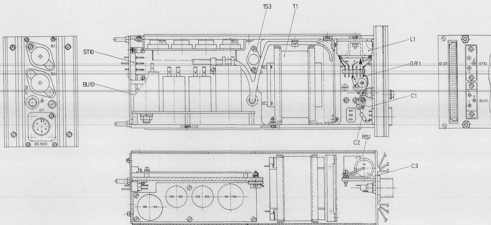
Batteriestromversorgung BS 1600 52.1817..000.00 (02)
