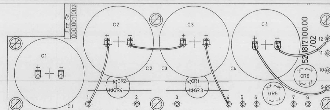
Elko-Aufbau 52.1817.100.00 (03)
