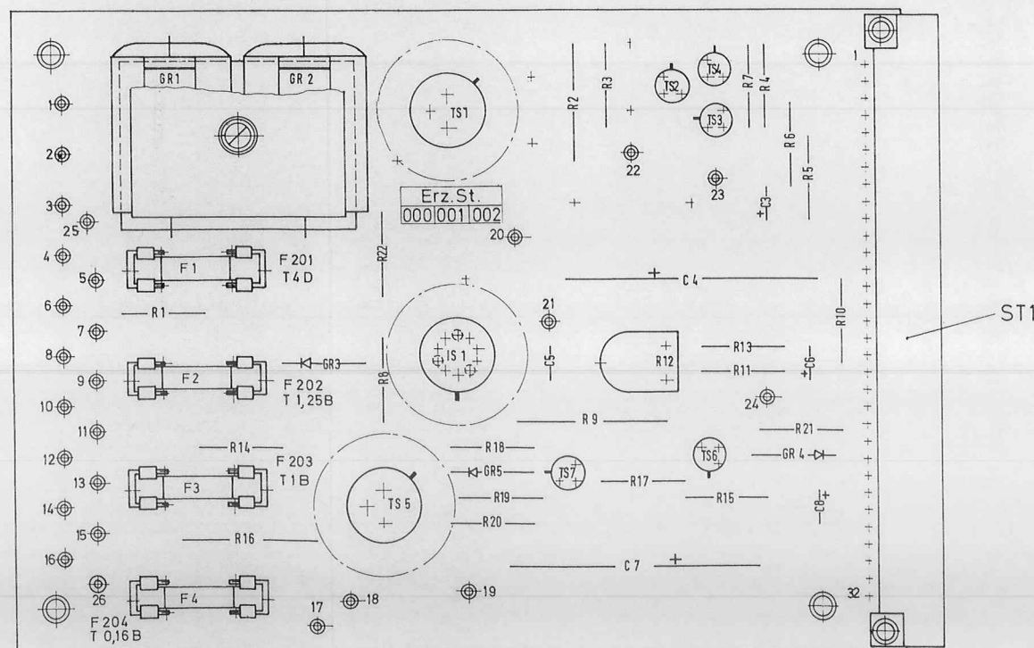
Stabilisierung 52.1817.200.00 (03)
