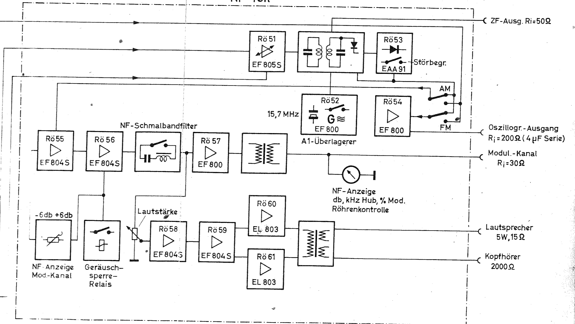
Bild 11. Blockschaltbild
