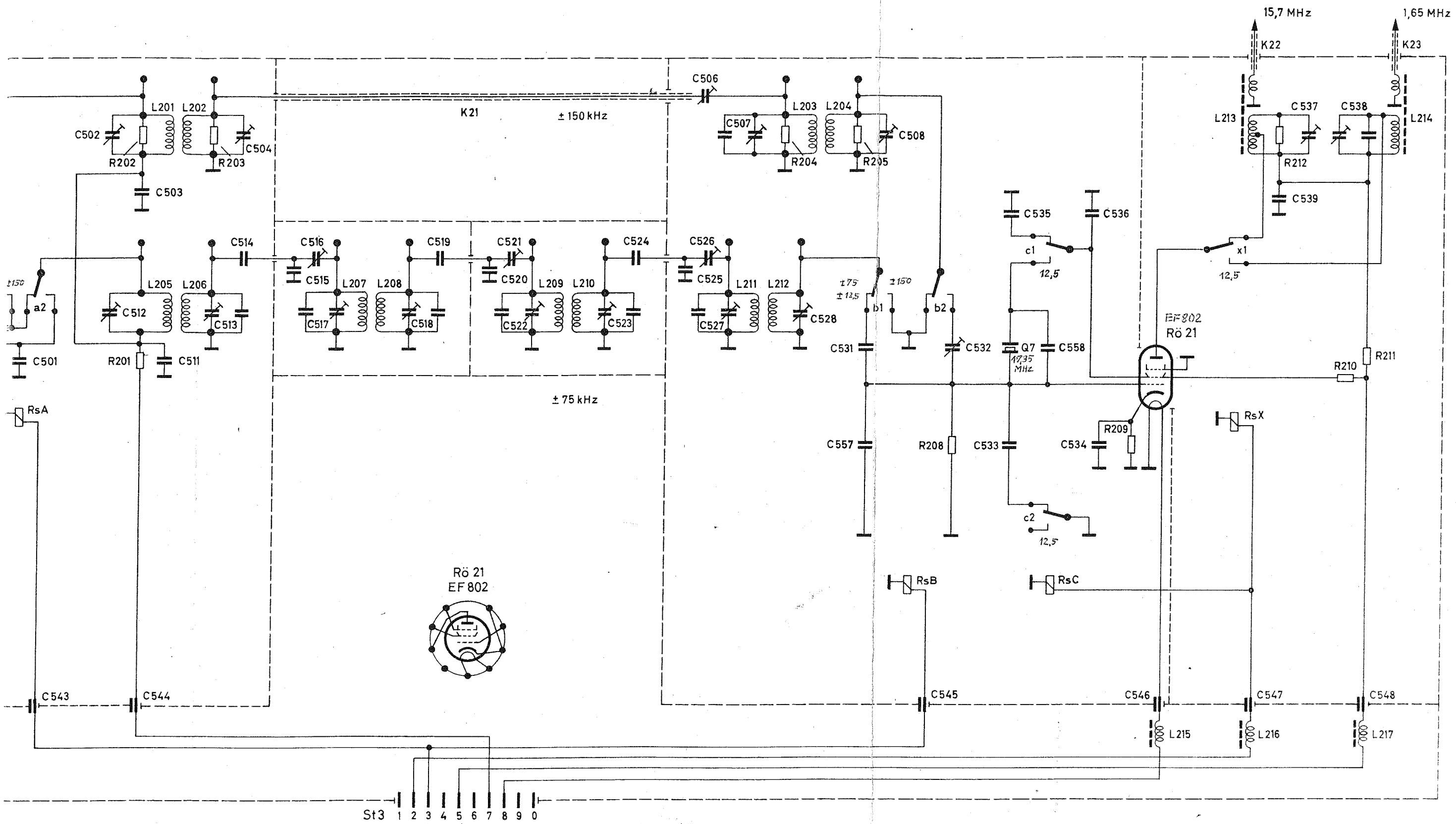
Bild 47. Stromlauf des ZF-Teiles I
