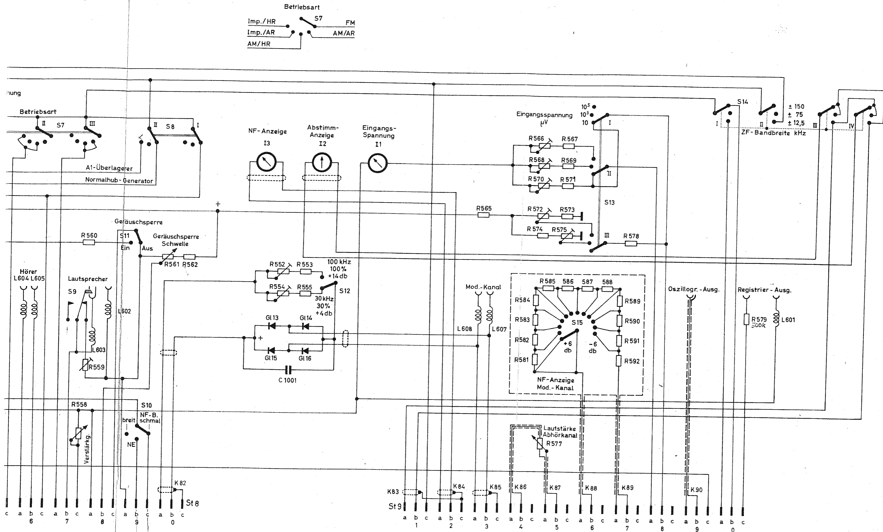
Bild 51. Stromlauf der Frontplatte
