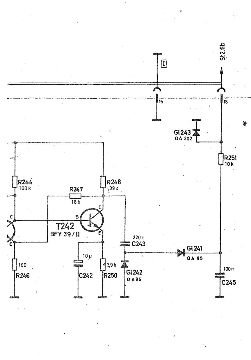
Synchron-Anzeige-Verstärker
