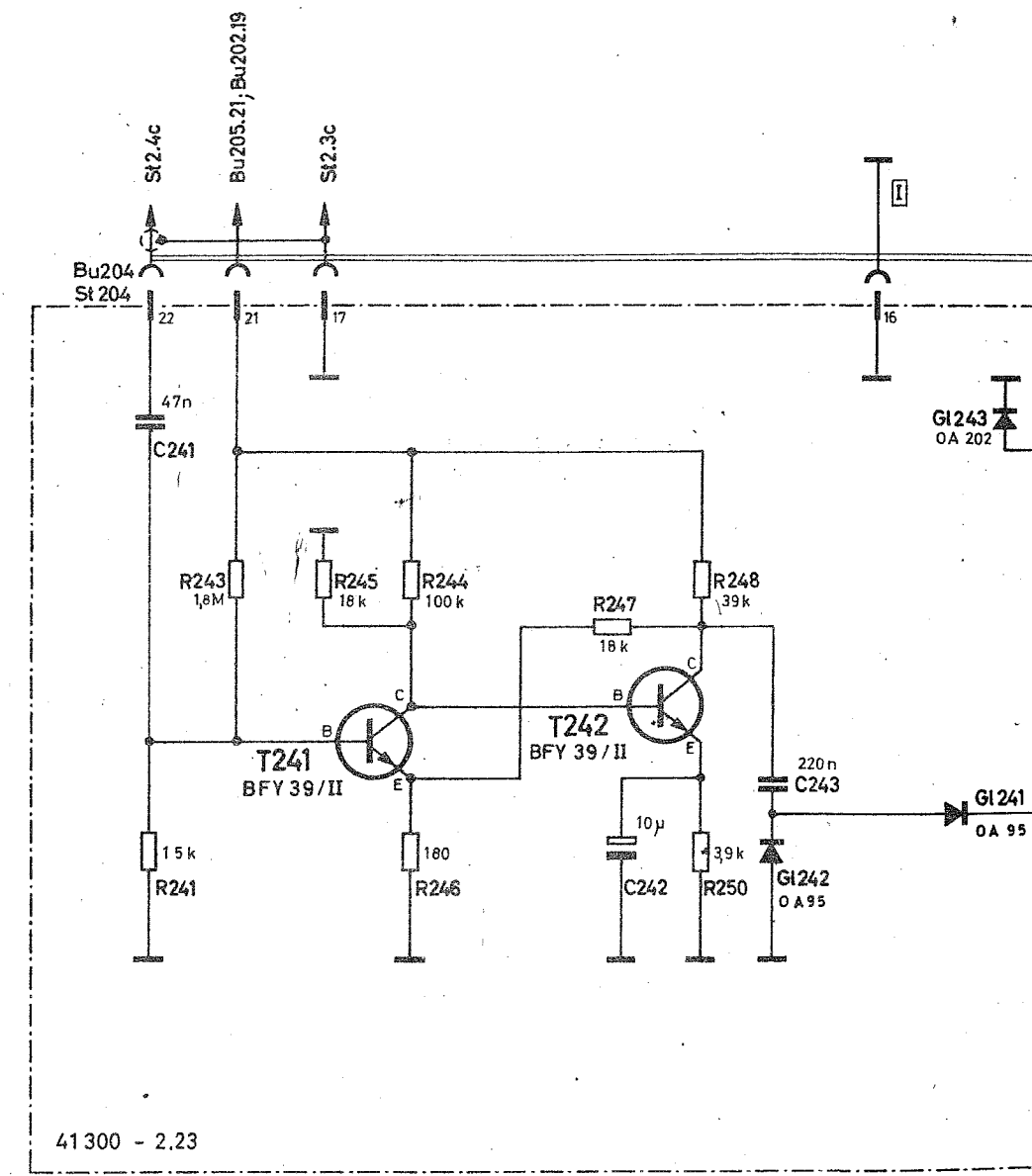
Synchron-Anzeige-Verstärker
