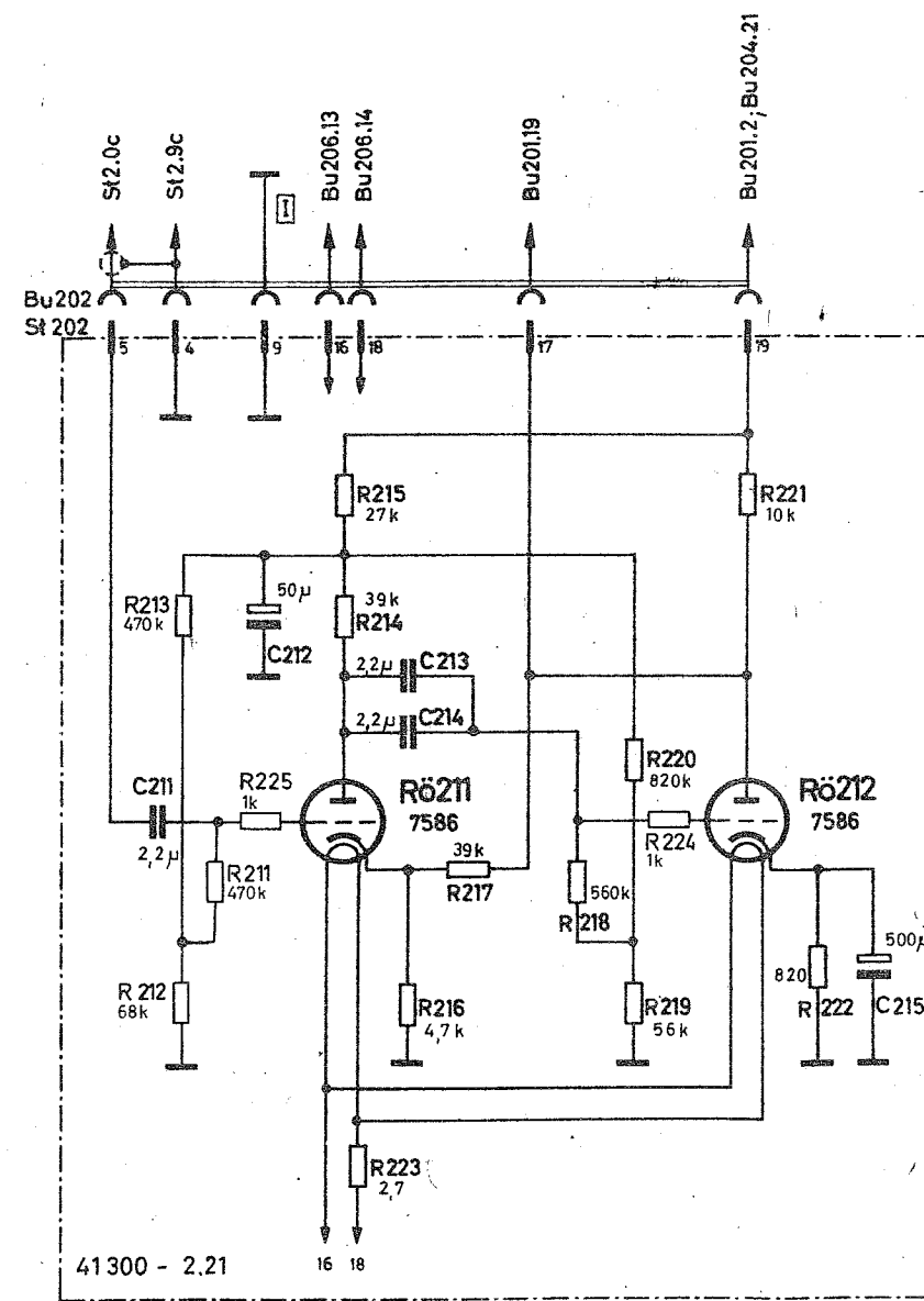
FM-Verstärker
