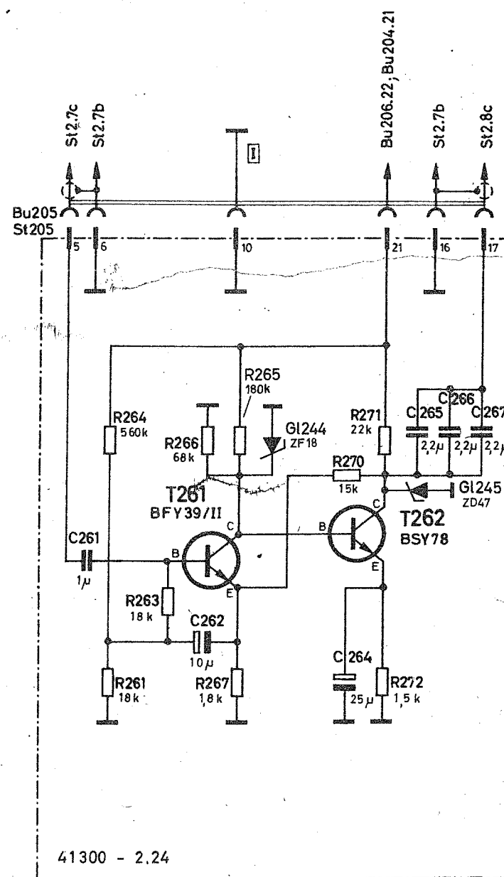
AM-Verstärker
