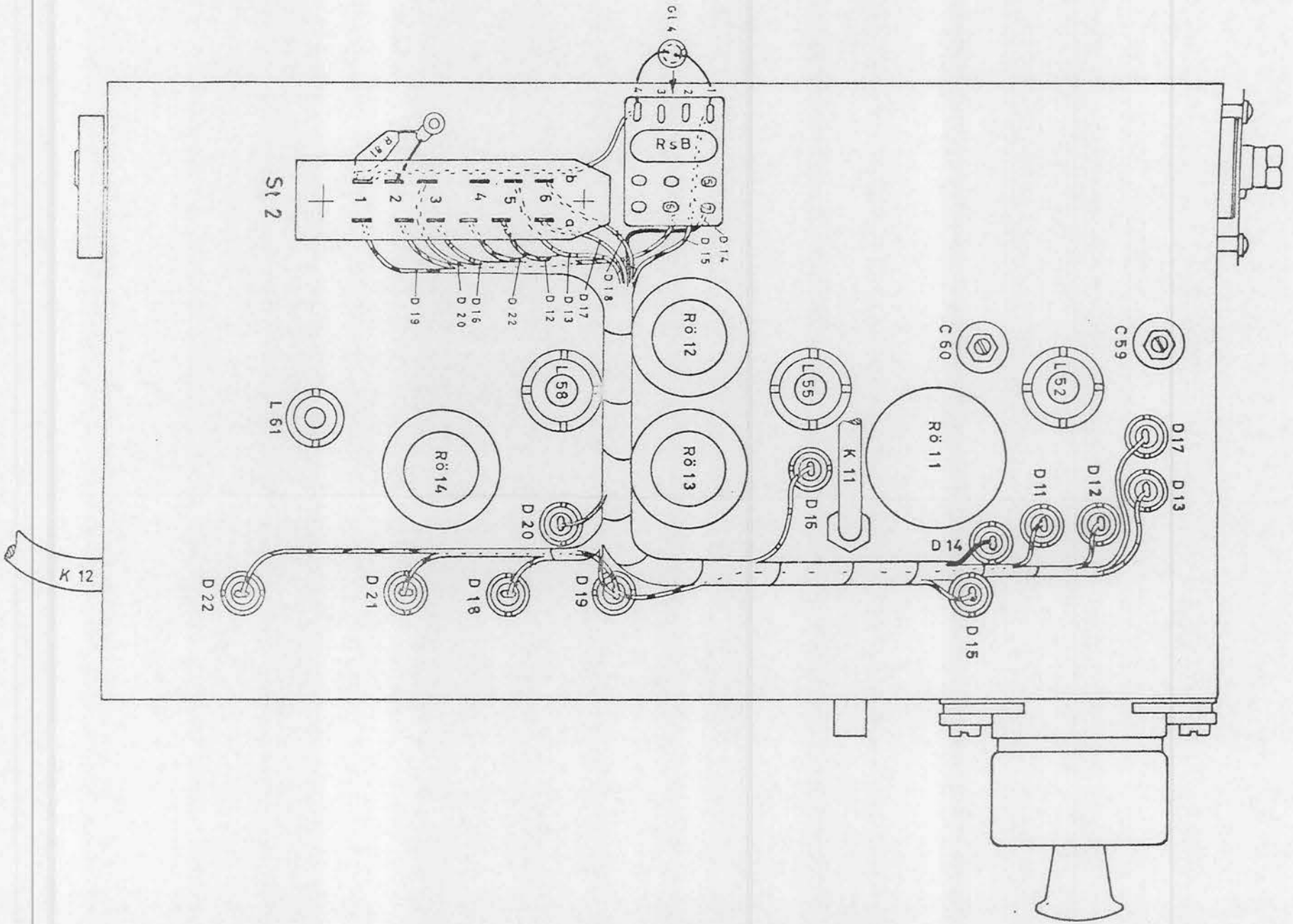
Positionierungsplan Versachsfacher
