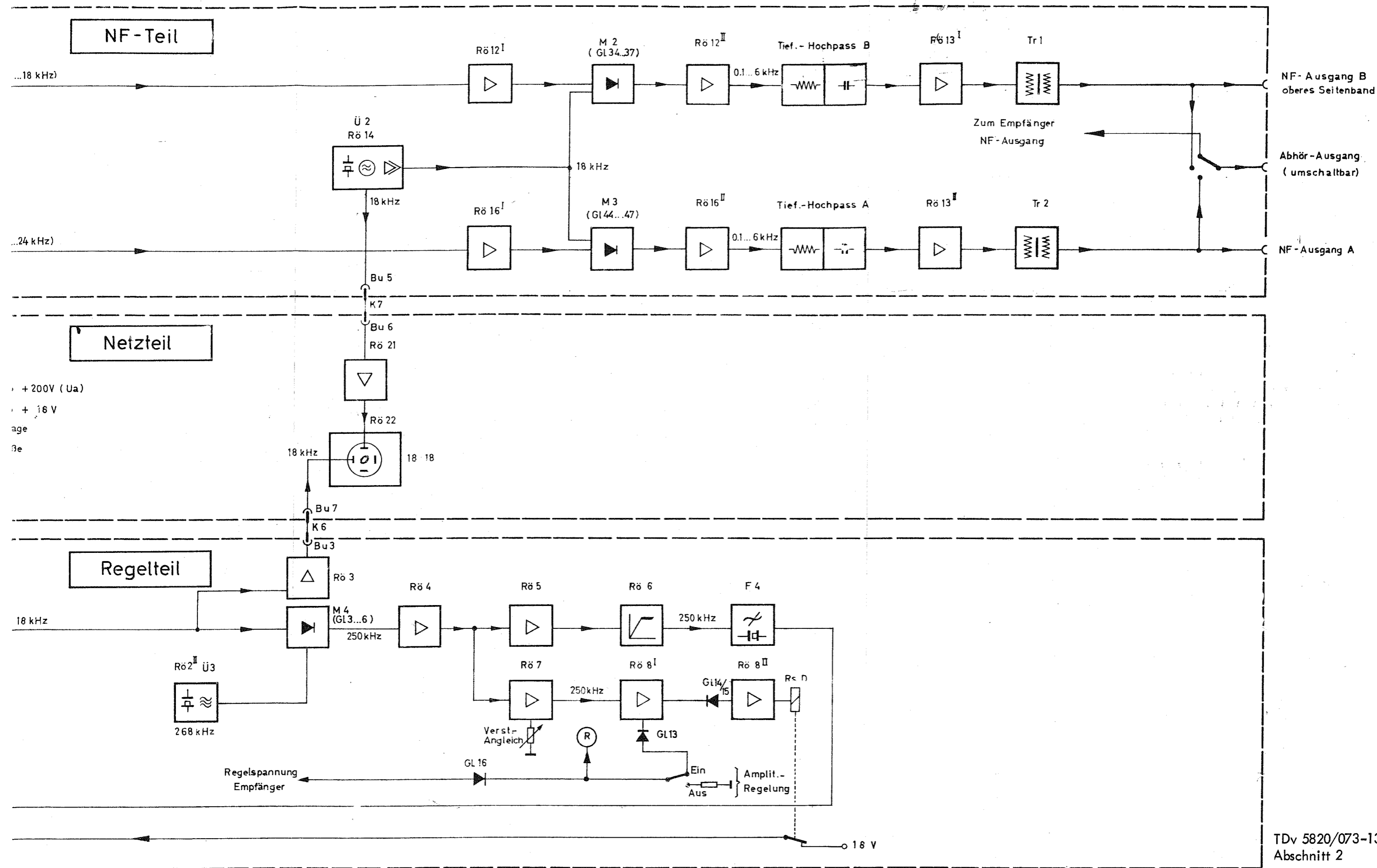
Blockschaltbild
