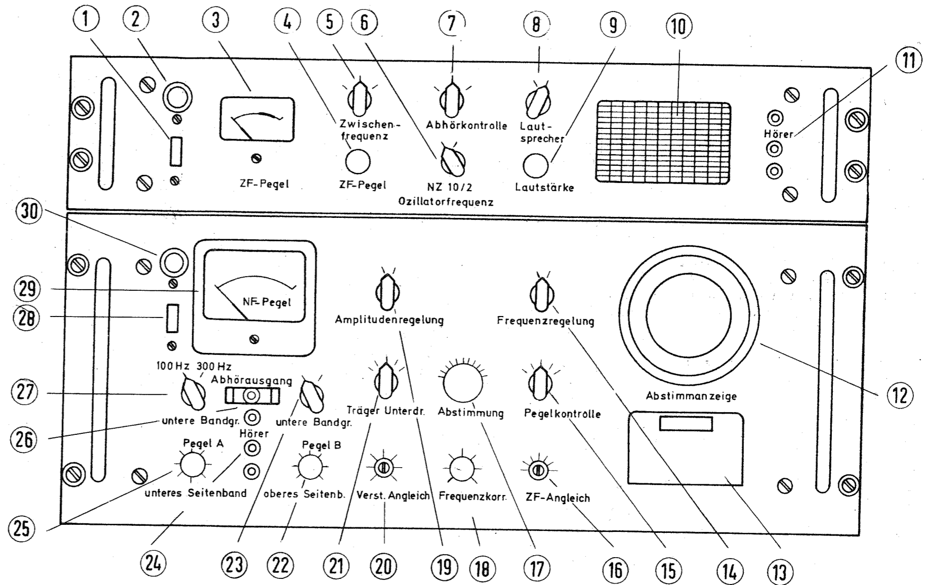
Bild 2 Bedienbild
