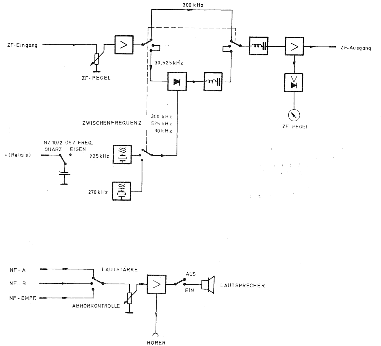
Bild 1 Blockschaftbild
