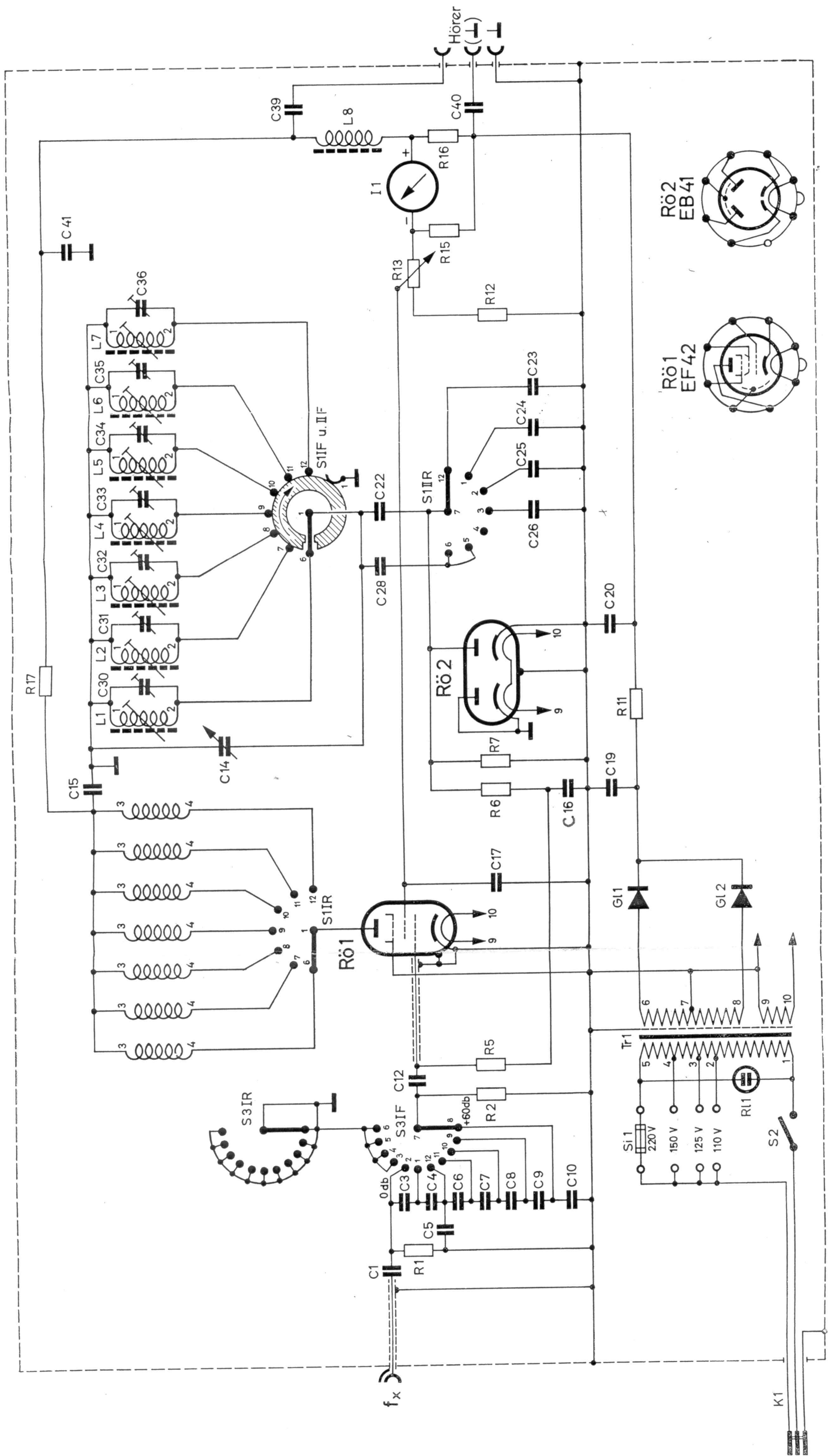
Bild 2. Stromlauf des Frequenzmessers Type WEN BN 435
